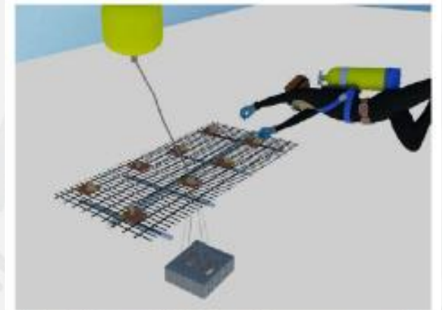
Ilustración 1. modelo de vivero tipo mesa suspendido multiple, diseño propio
